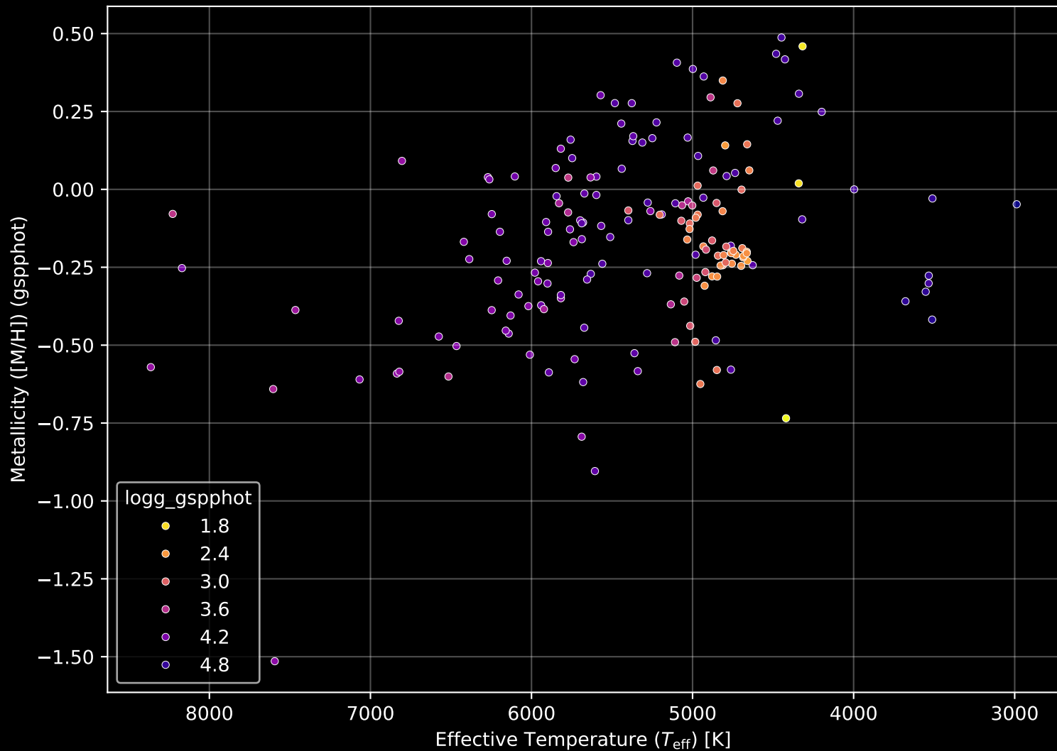
APOGEE DR17 Field: [CVZTILE_098+34_btx] Stellar Population Parameters (n= 176)
